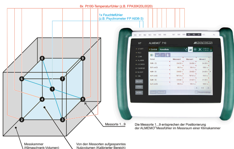
ALMEMO®-Setup zur Umsetzung der Richtlinie DAkkS-DKD-R 5-7 „Kalibrierung von Klimaschränken“
