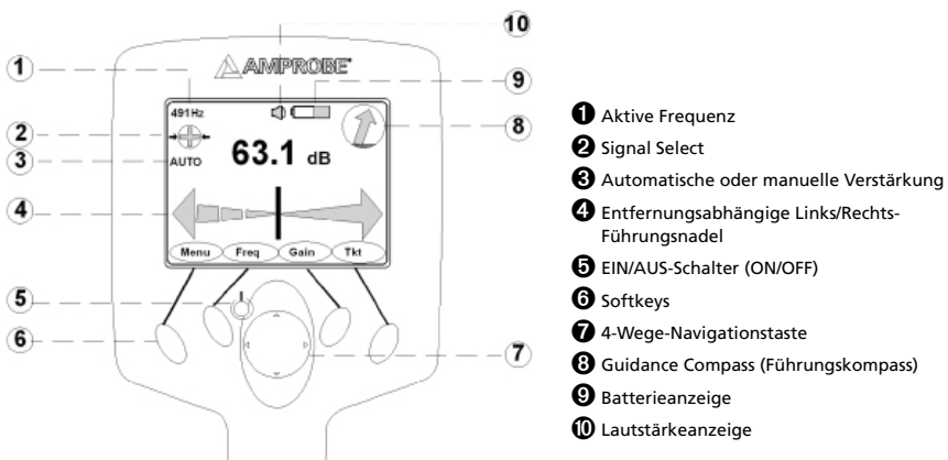
R-5000 Bedienungsfläche
