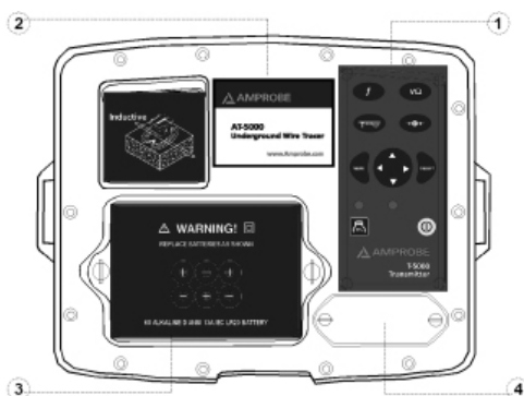
Vue de la face supérieure du T-5000
