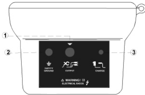
Vista del pannello laterale del trasmettitore T-5000
