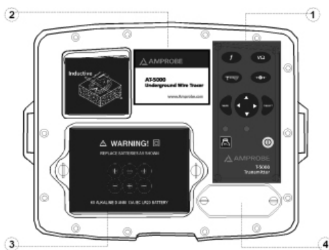
T-5000:s övre panel
