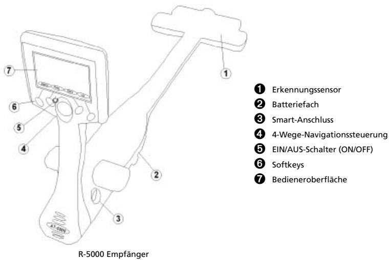
R-5000 Empfänger
