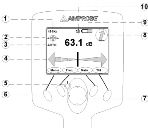
R-5000 driftsgränssnitt
