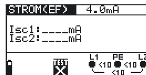
Abbildung 11.4: Messmenü für Fehlerstrom im Falle des ersten Fehlers
