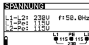
Abbildung 11.2: Beispiel für Spannungs- und Frequenzmessungen
