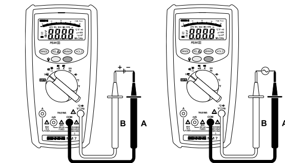
Bild 2: Gleichspannungsmessung Fig. 2: Direct voltage measurement Fig. 2: Mesure de tension continue Fig. 2: Meten van gelijkspanning Fig. 2: Medición de tensión continua Fig. 2: Likspänningsmätning σχήμα 2: μέτρηση DC-τάσης ill. 2: Misura tensione continua
