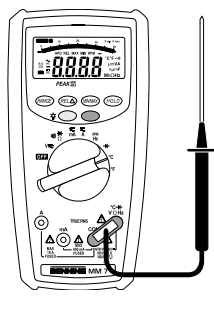
Bild 11: Temperaturmessung Fig. 11: Temperature measurement Fig. 11: Mesure de température Fig. 11: Meten van temperatuur Fig. 11: Medición de temperatura Fig. 11: Temperaturmätning σχήμα 11: Μέτρηση θερμοκρασίας ill. 11: Misura di temperatura
