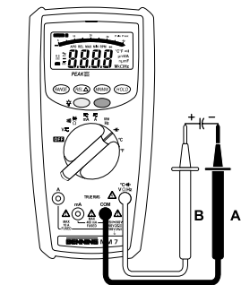
Bild 9: Kapazitätssmessung Fig. 9: Capacity Testing Fig. 9: Mesure de capacité Fig. 9: Capaciteitsmeting Fig. 9: Medición de capacidad Fig. 9: Kapacitansmätning σχήμα 9: Μέτρηση χωρητικότητας ill. 9: Misura di capacità
