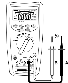
Bild 10: Frequenzmessung Fig. 10: Frequency measurement Fig. 10: Mesure de fréquence Fig. 10: Frequentiemeting Fig. 10: Medición de frecuencia Fig. 10: Frekvensmätning σχήμα 10: Μέτρηση συχνότητας ill. 10: Misura di frequenza
