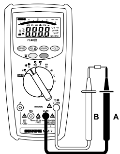
Bild 6: Widerstandsmessung Fig. 6: Resistance measurement Fig. 6: Mesure de résistance Fig. 6: Weerstandsmeting Fig. 6: Medición de resistencia Fig. 6: Resistansmätning σχήμα 6: Μέτρηση αντίστασης ill. 6: Misura di resistenza
