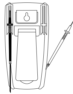
Bild 14: Aufwicklung der Sicherheitsmessleitung Fig. 14: Wrapping up the safety test leads Fig. 14: Enroulement du câble de mesure de sécurité Fig. 14: Wikkeling van veiligheidsmeet snoeren Fig. 14: Arrollamiento de la conducción protegida de medición Fig. 14: Placering av säkerhetsmåtsladdar σχήμα 14: Τυλίξτε τα καλώδια μέτρησης ill. 14: Avvolgimento dei cavetti di sicurezza
