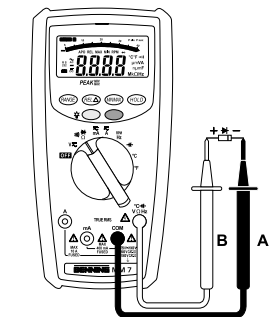
Bild 7: Diodenprüfung Fig. 7: Diode Testing Fig. 7: Contrôle de diodes Fig. 7: Diodecontrole Fig. 7: Verificación de diodos Fig. 7: Diod-test σχήμα 7: Έλεγχος διόδου ill. 7: Prova diodi
