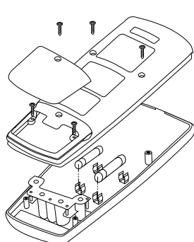
Bild 13: Sicherungswechsel Fig. 13: Fuse replacement Fig. 13: Remplacement des fusibles Fig. 13: Vervanging van de smeltzekeringen Fig. 13: Cambio de fusible Fig. 13: Säkringsbyte σχήμα 13: αντικατάσταση μπουσάριας ill. 13: Sostituzione fusibile
