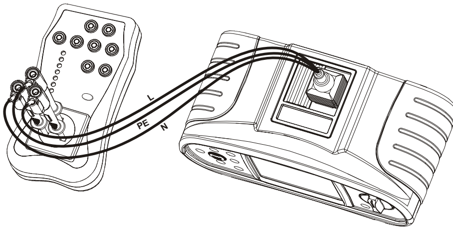
Abb. 4.2:: Durchführung der Fehlerschleifenimpedanzkalibrierung mit dem Universalprüfkabel
