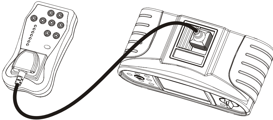
Abb. 4.1:: Durchführung der Fehlerschleifenimpedanzkalibrierung mit dem Steckerkabel
