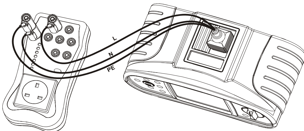
Abb. 4.3.: Durchführung der Kalibrierung der Isolationswiderstands-Funktion mit dem Universalprüfkabel
