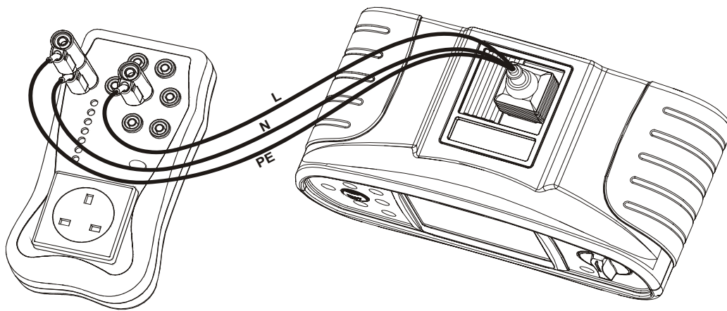
Abb. 4.4.: Performing low resistance calibration using universal test cable Durchführung der Kalibrierung der Niederohm-Funktion mit dem Universalprüfkabel
