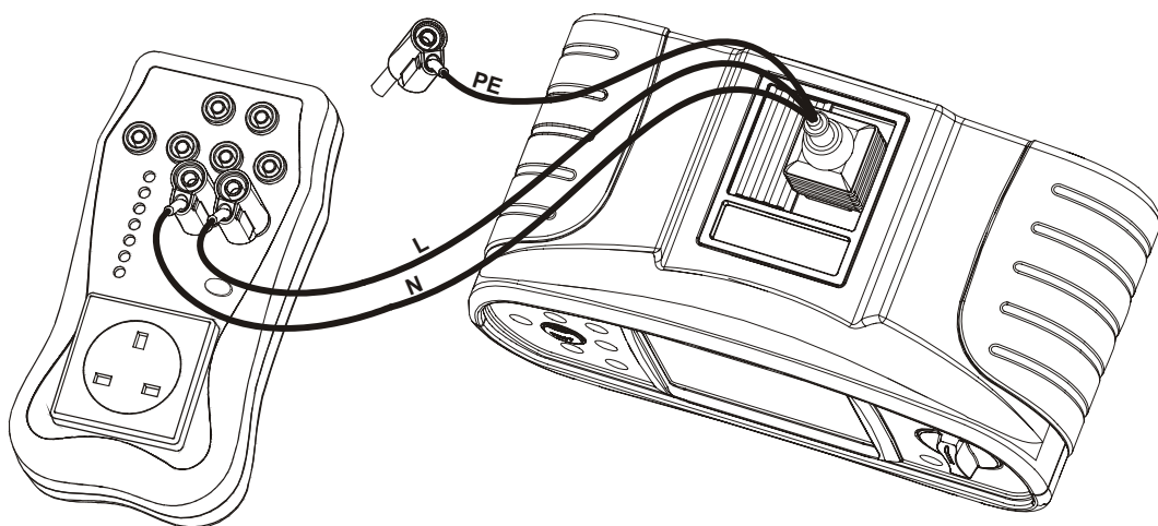
Abb. 4.5: Durchführung der Spannungs- und Frequenzkalibrierung mit dem Universalprüfkabel
