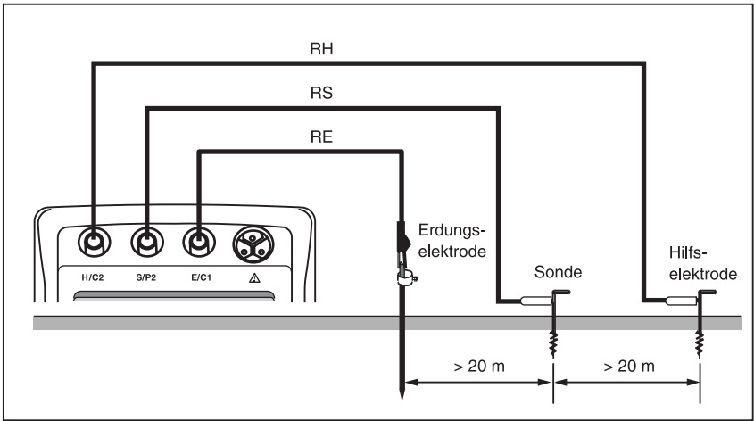
Abbildung 4. Messanordnung 3-Pol-Messung
