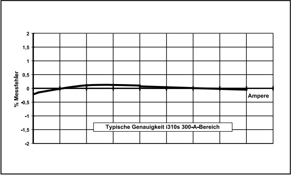
Typische Genauigkeit
