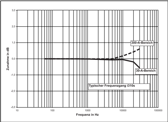
Typischer Frequenzgang
