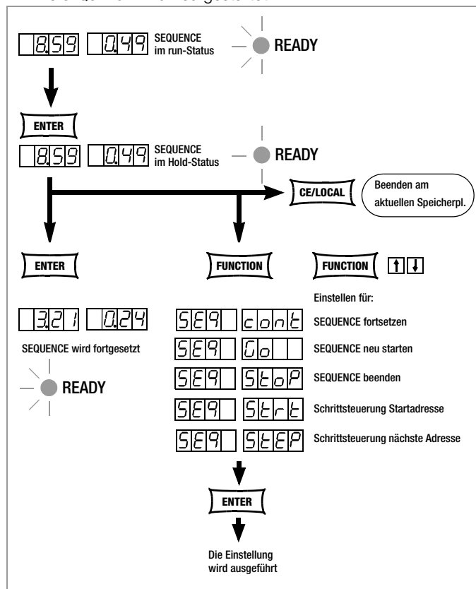
Bild 4.7.3 j Anhalten und Fortsetzen einer SEQUENCE
