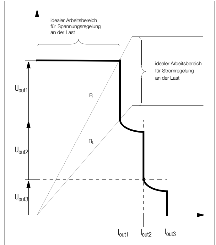
Bild 5.9.1b U / I-Diagramm bei direkter Serienschaltung
