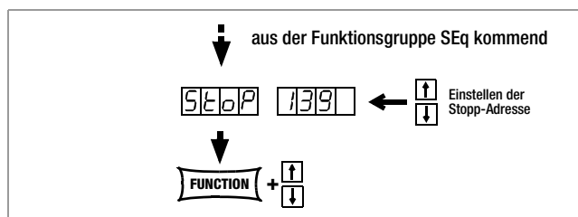
Bild 4.7.3 e Weg zur Einstellung der Stopp-Adresse
