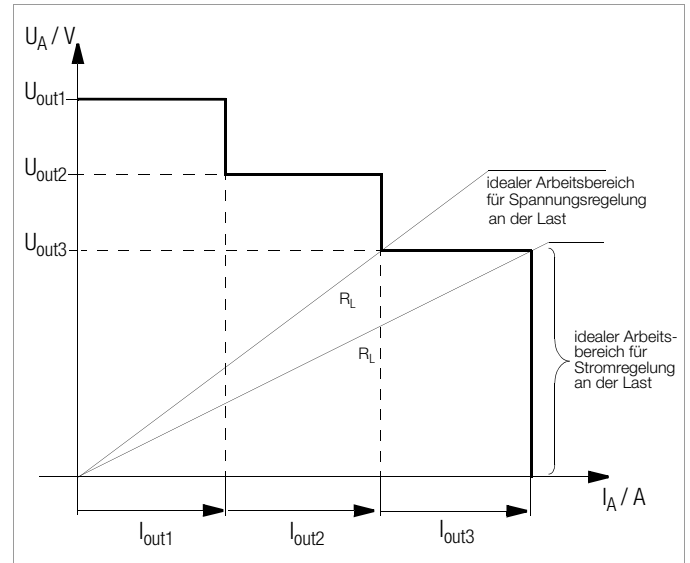
Bild 5.8.1b U / I-Diagramm bei direkter Parallelschaltung
