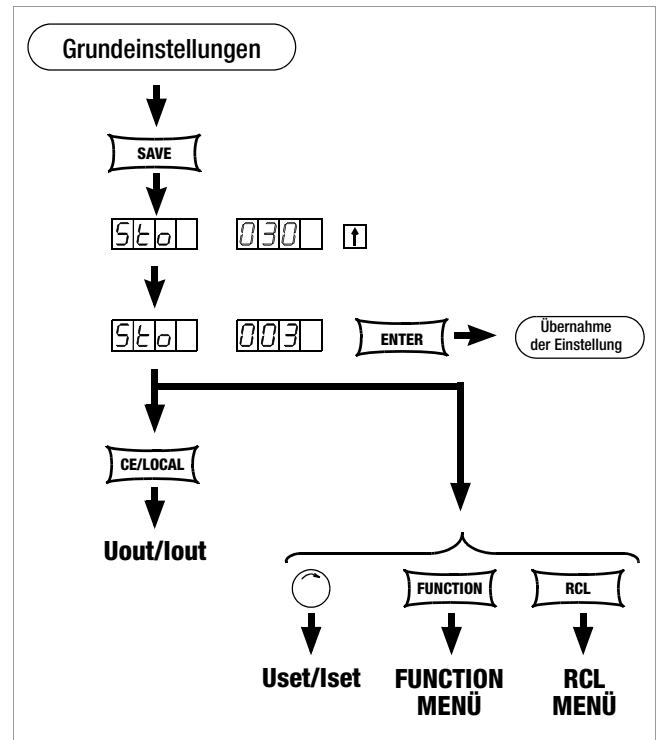
Bild 4.10.1 Speichern der Geräteeinstellung
