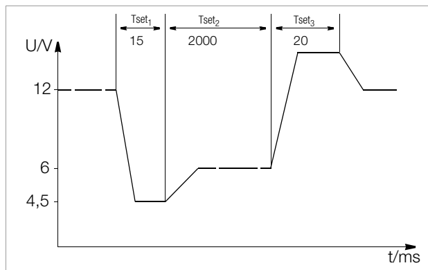
Bild 4.7.3 Prüfsignal zur Bordnetz-Simulation beim Anlassvorgang
