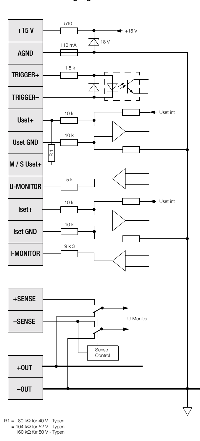
Bild 5.1 Fühlerbetrieb
