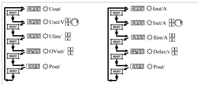
Bild 4.8.1 Anzeigenumschaltung mit der SELECT-Taste
