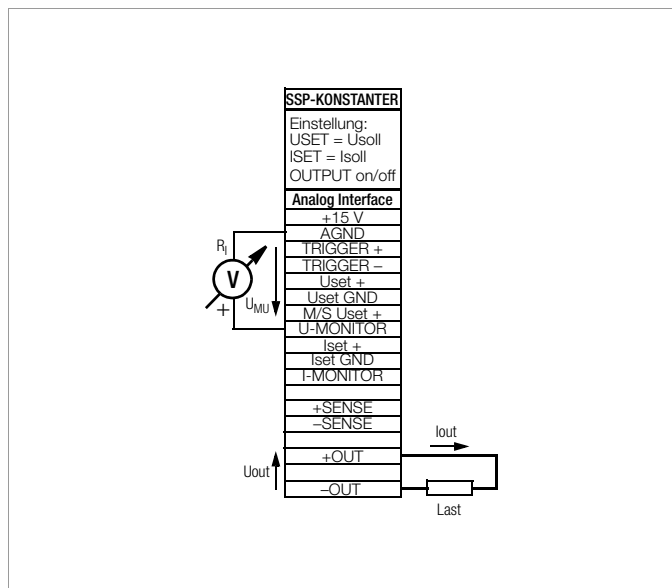
Bild 5.5 Verdrahtung Spannungsmonitor
