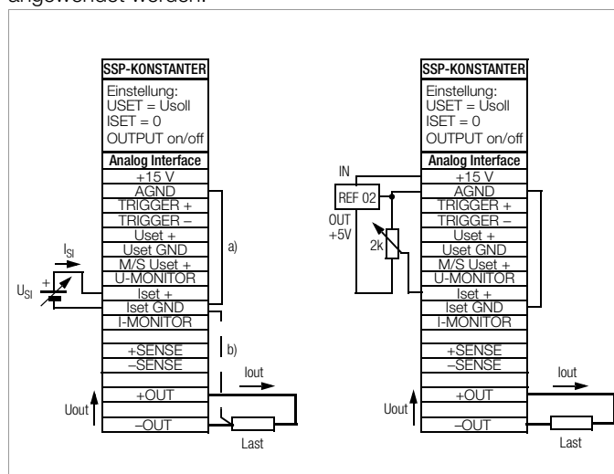
Bild 5.4a Verdrahtung für Stromsteuerung durch externe Spannung
