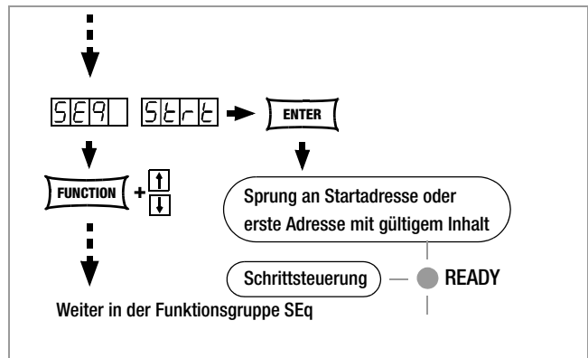
Bild 4.7.3 g Vorbereiten einer Schrittsteuerung
