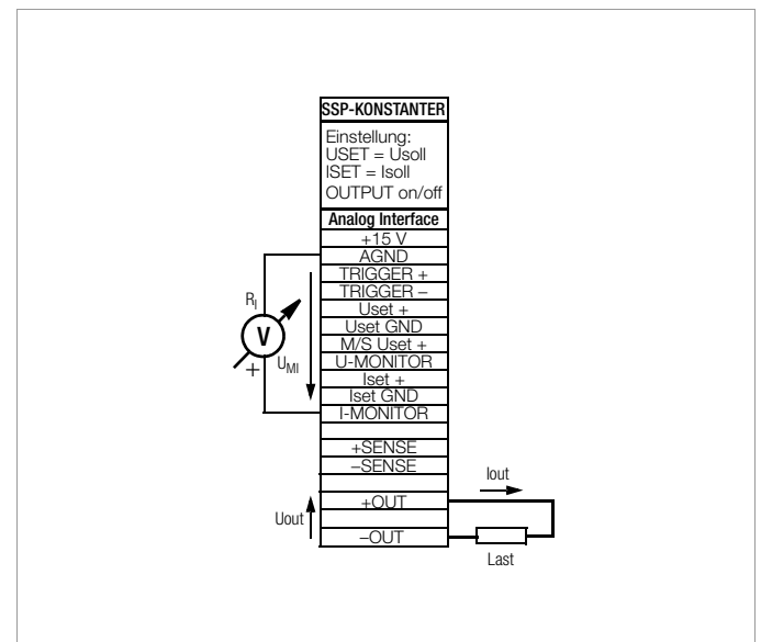
Bild 5.6 Verdrahtung Strommonitor
