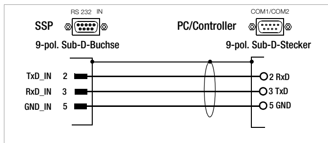
Bild 1.5.2 Verbindungskabel für serielle Schnittstelle
