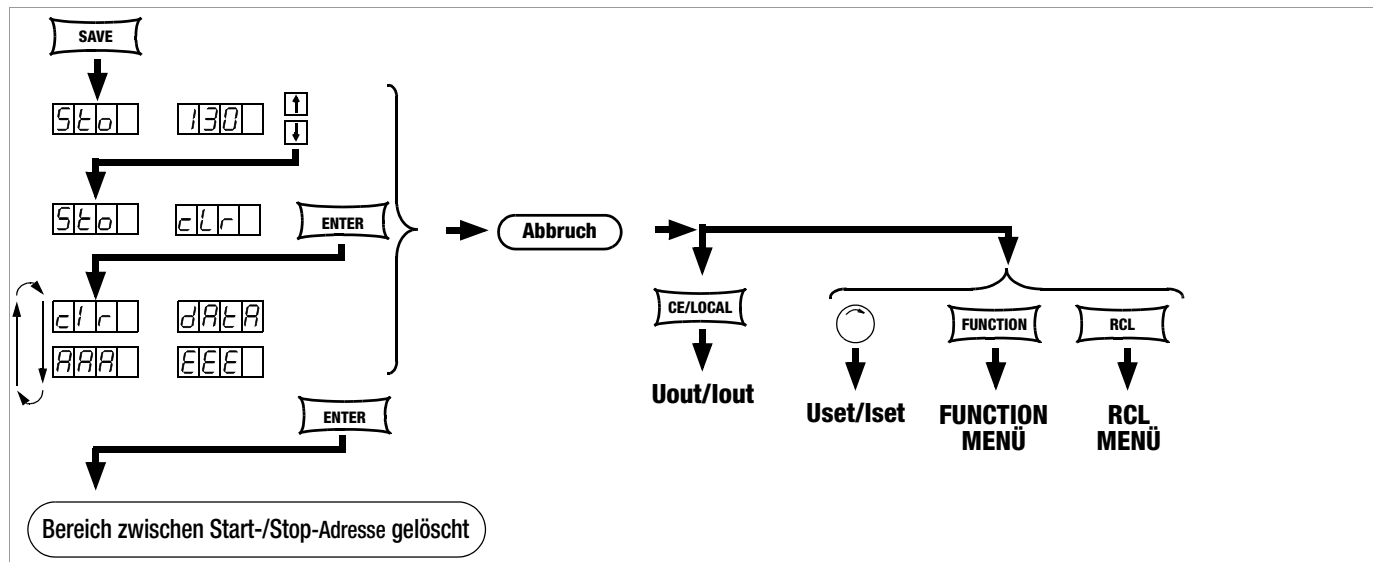
Bild 4.10.3 Löschen aller Inhalte zwischen Start-/Stopp-Adresse
