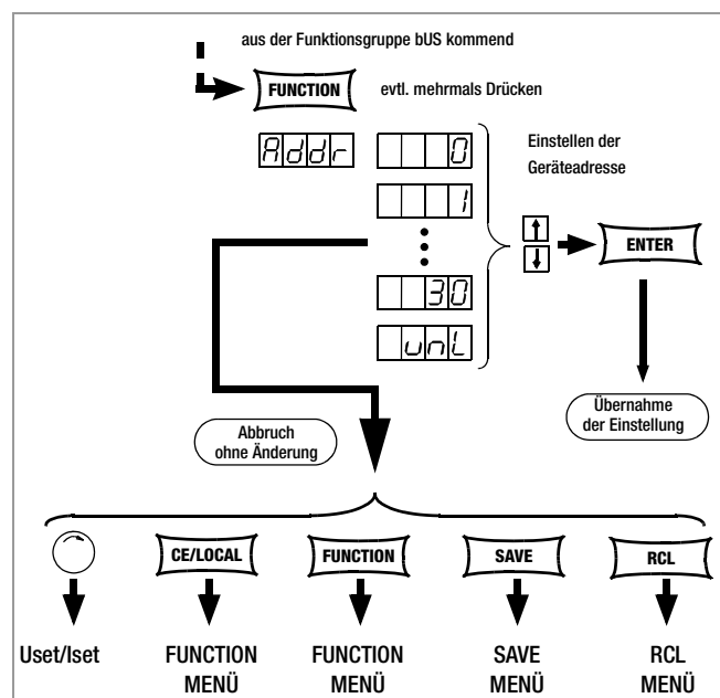
Bild 4.7.4 a Weg zur Einstellen der Geräte-Adresse
