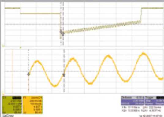
Erzeugung eines Spannungsverlaufs der Kfz-Bordspannung beim Starten des Motors.
