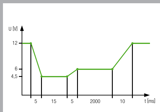
Oszillogramm der SYSKON-Ausgangsspannung - Anlasserkurve mit steigendem Sinus. Sinusfunktion als Unterprogramm im Ablauf eingebunden.
