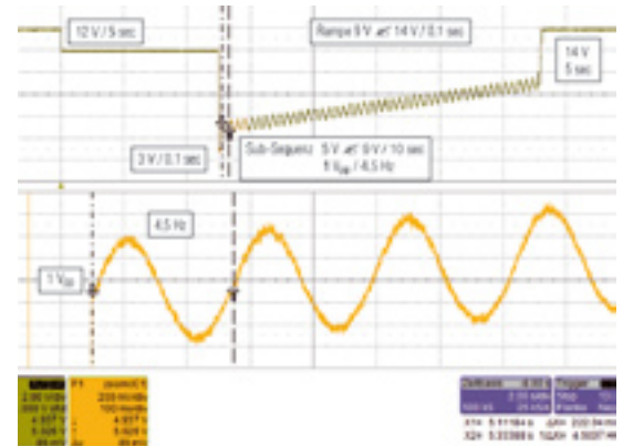
Erzeugen einer Kfz-Anlasserkennlinie
