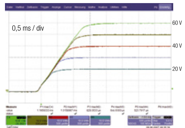
Anstiegszeit der eingestellten Nenn-Leistung
