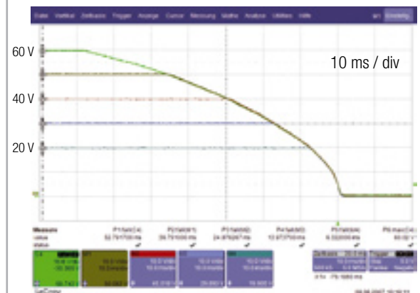
Abstiegszeit der eingestellten Nenn-Leistung
