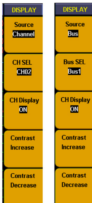
Fig 76: Display menu
