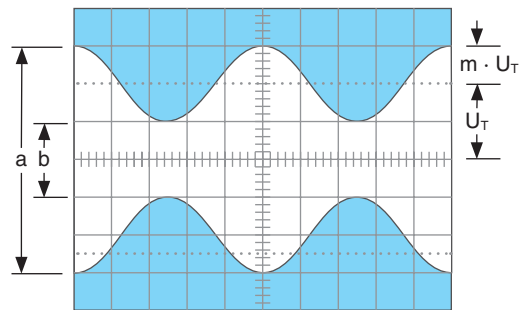
Abb. 2 Amplitudenmodulierte Schwingung: F = 1 MHz; f = 1 kHz; m = 50\% ; U_T = 28,3 mV eff .
