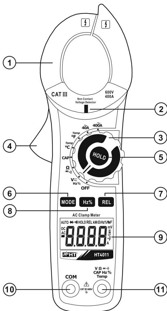
Abb. 1: Gerätebeschreibung
