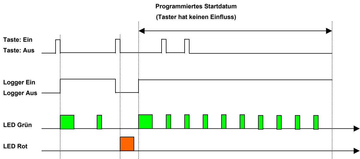
Timing Diagram: Datenlogger THC/TIC im Start/Stop-Modus
