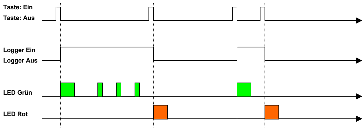
Timing Diagram: Datenlogger THC/TIC im Ring-Modus
