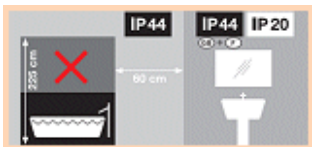
Schutzonen im Bad
