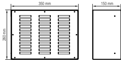
Schalldämm-Modul
