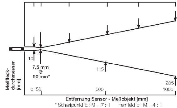
Scharfpunktoptik OS2
