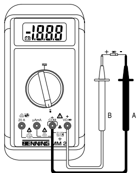
Bild 7: Diodenprüfung Fig. 7: Diode Testing Fig. 7: Contrôle de diodes Fig. 7: Diodcontrole Fig. 7: Verificación de diodos Fig. 7: Diod-test ill. 7: Prova diodi
