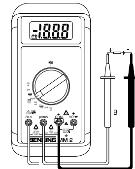
Bild 4: Gleichstrommessung Fig. 4: DC current measurement Fig. 4: Mesure de courant continu Fig. 4: Meten van gelijkstroom Fig. 4: Medición de corriente continua Fig. 4: Resistansmätning ill. 4: Misura corrente continua
