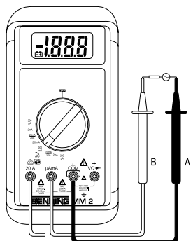
Bild 5: Wechselstrommessung Fig. 5: AC current measurement Fig. 5: Mesure de courant alternatif Fig. 5: Meten van wisselstroom Fig. 5: Medición de corriente alterna Fig. 5: Genomgångstest med summer ill. 5: Misura corrente alternata
