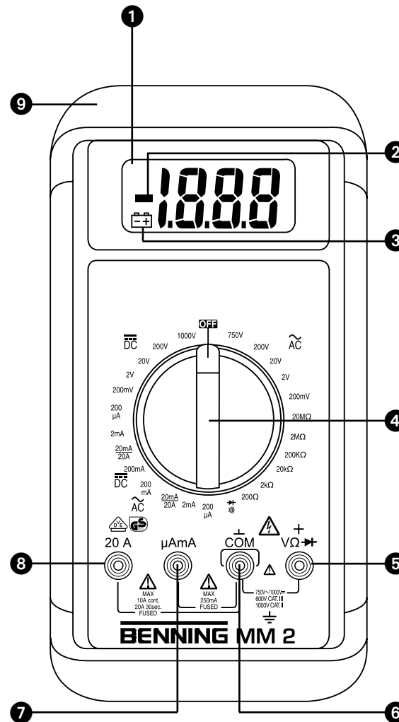
Bild 1: Gerätefrontseite Fig. 1: Front tester panel Fig. 1: Panneau avant de l'appareil Fig. 1: Voorzijde van het apparaat Fig. 1: Parte frontal del equipo Fig. 1: Instrumentfront ill. 1: Lato anteriore apparecchio
