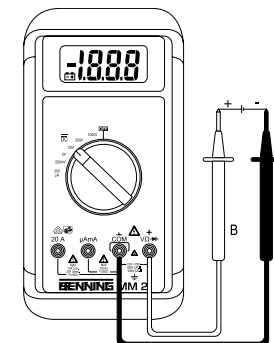
Bild 2: Gleichspannungsmessung Fig. 2: Direct voltage measurement Fig. 2: Mesure de tension continue Fig. 2: Meten van gelijkspanning Fig. 2: Medición de corriente continua Fig. 2: Likspänningsmätning ill. 2: Misura tensione continua
