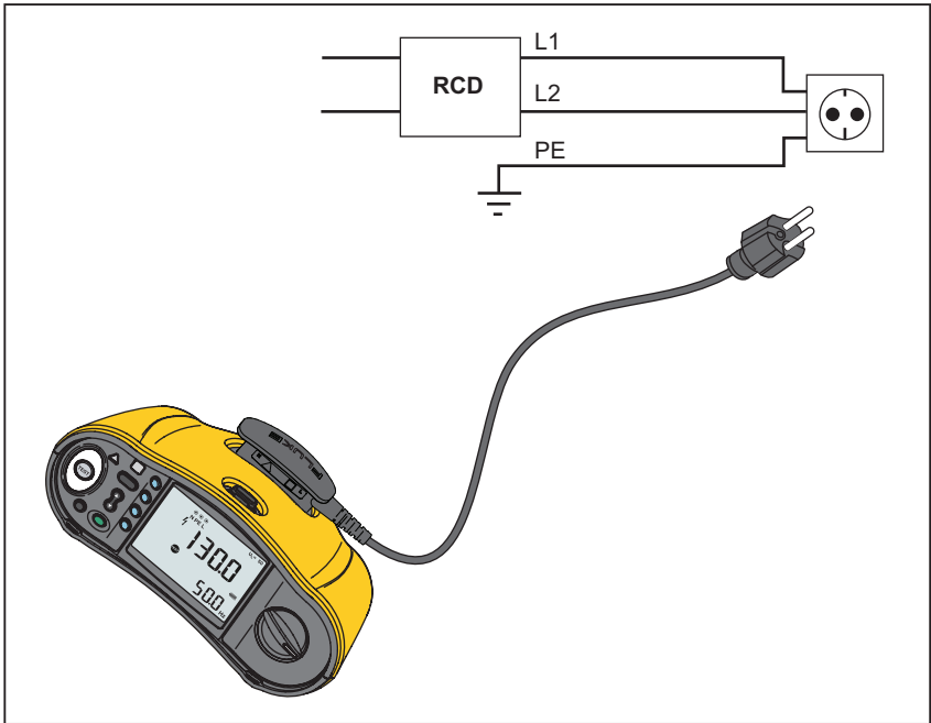
Abbildung 9. Konfiguration mit einzelner Prüfleitung
