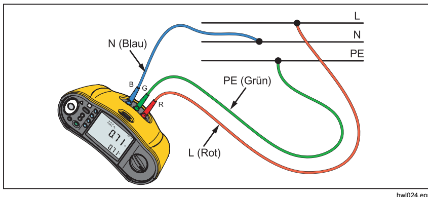
Abbildung 13. Dreikabelanschluss für Erdungswiderstand-Schleifenmessung (Auslösefreier Modus)
