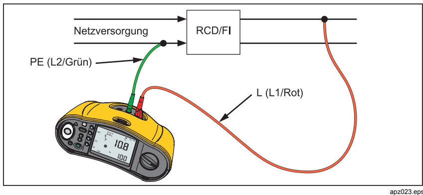
Abbildung 8. Verbindung für RCD/FI-Prüfung in Umgebungen mit IT-Systemen
