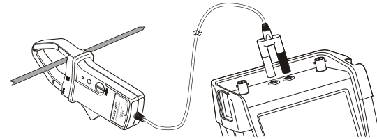
Abbildung 16. Meßanordnung
