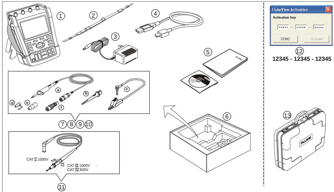
Abbildung 1. ScopeMeter-Messgerätsatz
