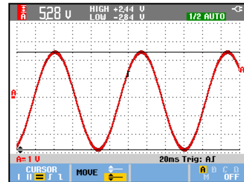
Abbildung 25. Spannungsmessung mit Hilfe der Cursors
