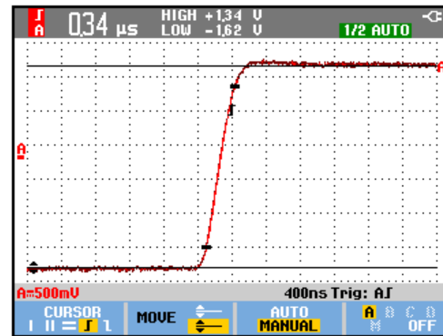
Abbildung 27. Anstiegszeitmessung
