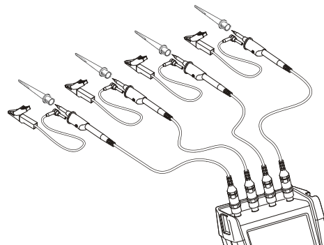
Abbildung 38. Elektronische Anschlüsse für Messungen mittels Hakenklemmen und Krokodilklemmen-Erdung
