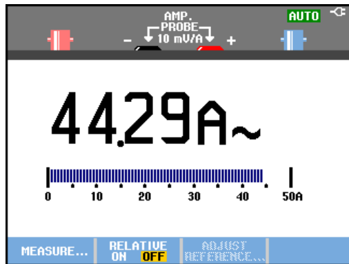
Abbildung 17. Stromstärken-Meßwerte
