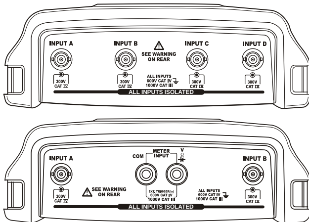
Abbildung 5. Messeingänge
