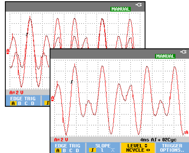
Abbildung 31. N-Zyklus-Triggerung
