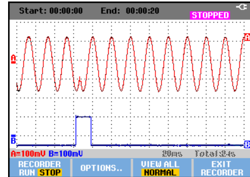
Abbildung 21. Aufzeichnen von Signalformen
