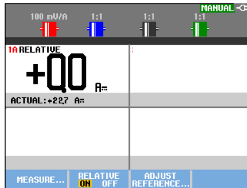
Abbildung 13. Durchführen einer Relativ-Messung
