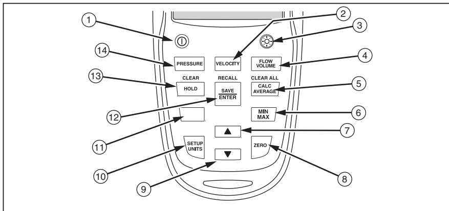
Abbildung 1. 922 Luftmengenmesser
