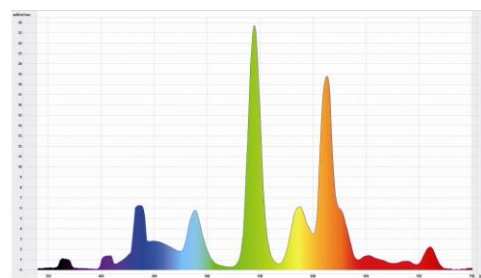
Linienspektrum Leuchtstoffröhre TL8 840
