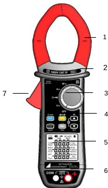
Abbildung 1 : Vielfachmesszange METRACLIP 87
