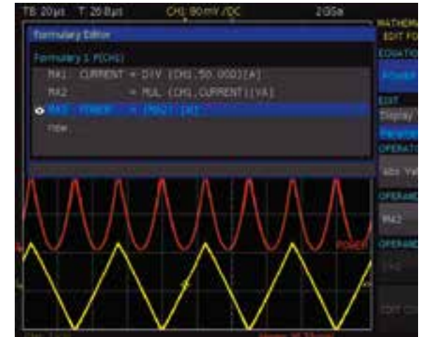
Formeleditor-Ansicht der komplexen Mathematikfunktion (R&S®HMO1202 Serie)
