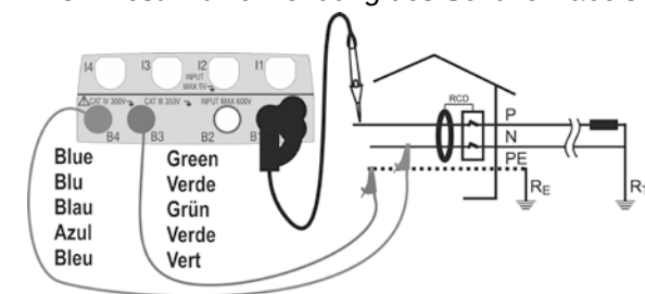
RCD Test mit Sonde PR400
