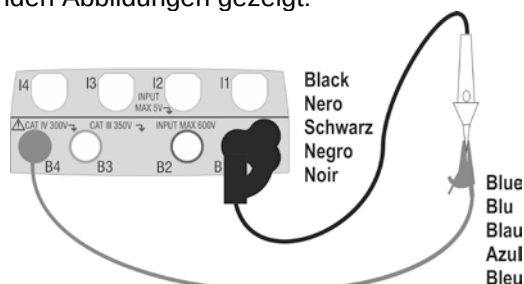
Kalibration mit der Prüfsonde PR400
