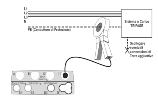
Messung des direkten Leckstromes bei drei Phasen
