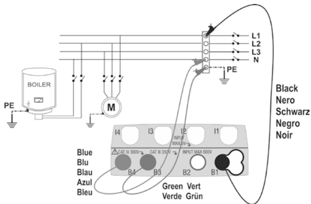
Isolationsmessung mit Einsatz der Messleitungen
