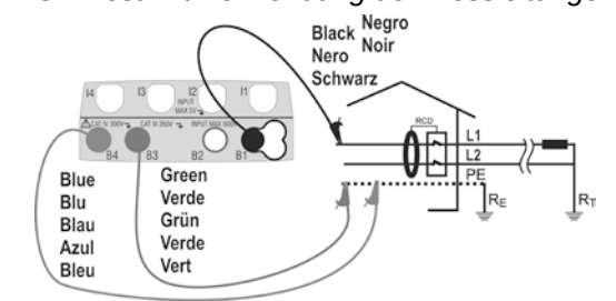
RCD Test in zweiphasigem System 230V ohne Neutralleiter
