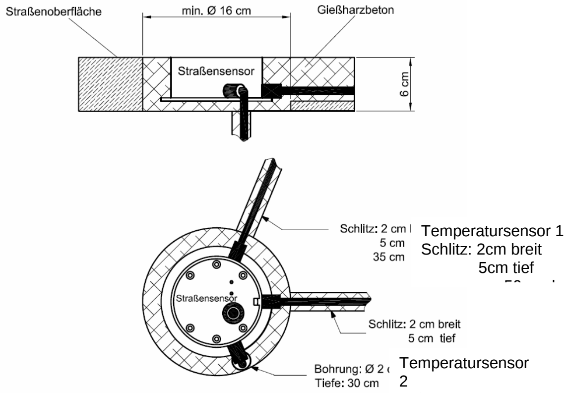
Abb. 2: IRS31 Einbau in der Straße bei 2 externen Temperaturfühlern
