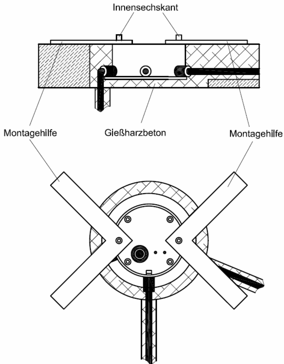
Abb. 3: Montage des IRS31
