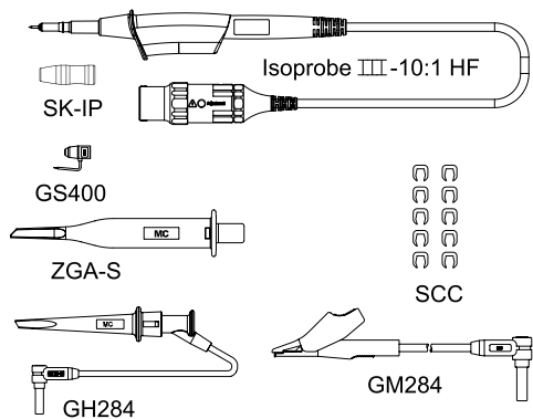
Lieferumfang / Supplied components / Composition du lot SET Isoprobe III-10:1 HF
